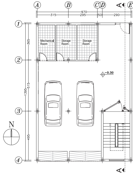
شکل ۴: نقشه پلان طبقه همکف
