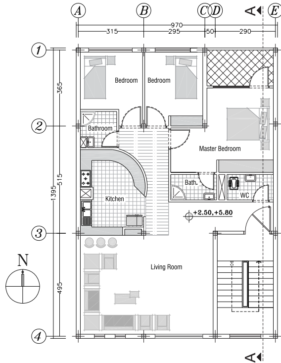
شکل ۳: نقشه پلان تیب طبقات
